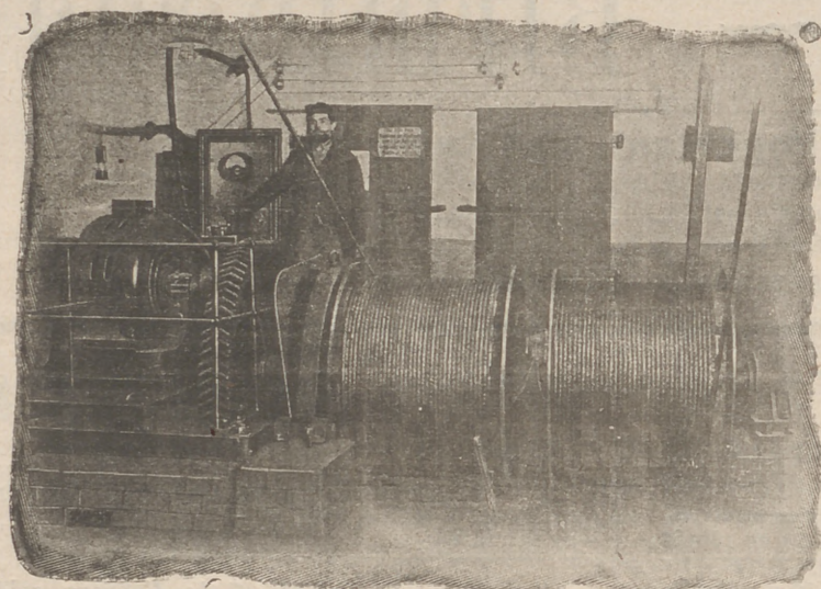
Torno doble para minas, movido por motor de corriente alterna trifásica
