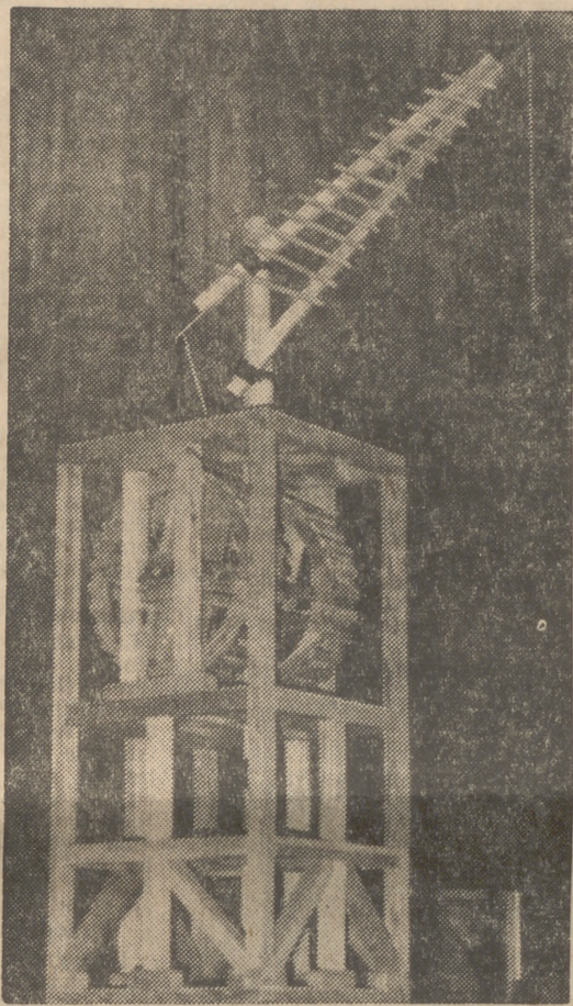
La pluma-grúa de Juan de Herrera es una de las maquetas de la muestra que hace evocar la riqueza de ideas de los antiguos inventores desprovistos de medios. Con ella, en tiempos de Felipe II, el arquitecto consiguió levantar el Monasterio de El Escorial
