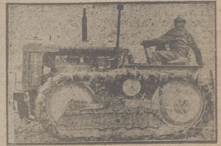
Ya conocemos el modelo Fordson semi-oruga. Hoy publicamos la última modificación efectuada en estos tractores y es la construcción de los mismos con oruga completa.
