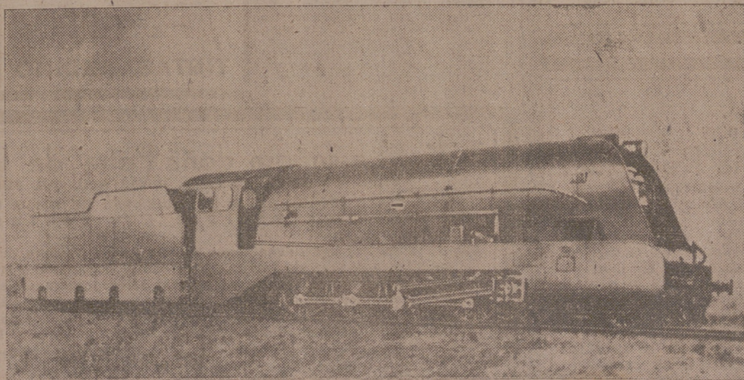
Las fábricas españolas están construyendo 750 locomotoras de los más modernos tipos. Pronto serán entregadas quince. Pesan 116 toneladas, desarrollan una velocidad de 110 kilómetros por hora y cuestan sesenta mil pesetas. Tanto el material, como la dirección y mano de obra, son totalmente españoles (Foto CIFRA)
