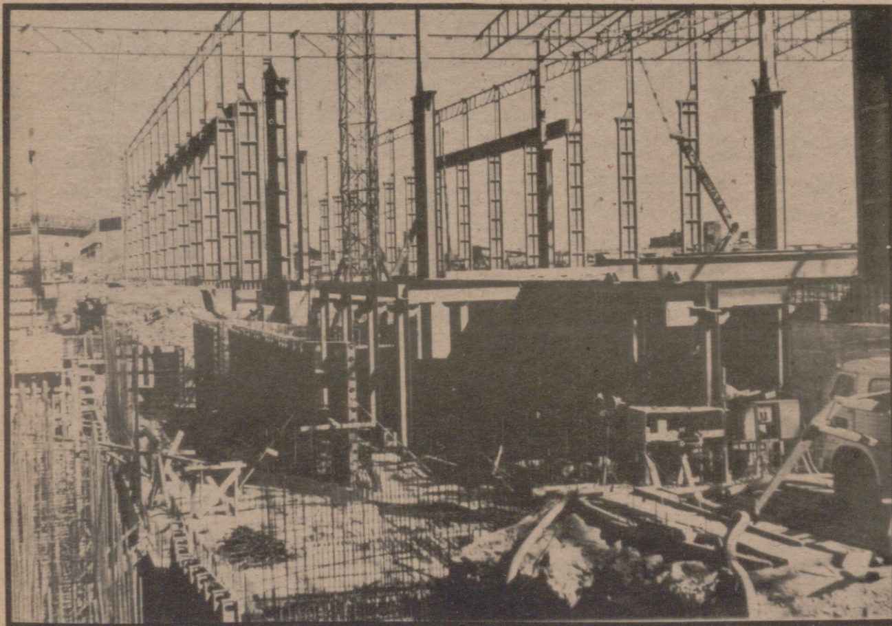
SAGUNTO (Valencia). Aspecto actual de las obras para la construcción de la cuarta planta siderúrgica de España en esta localidad valenciana (Foto Cifra Gráfica)
