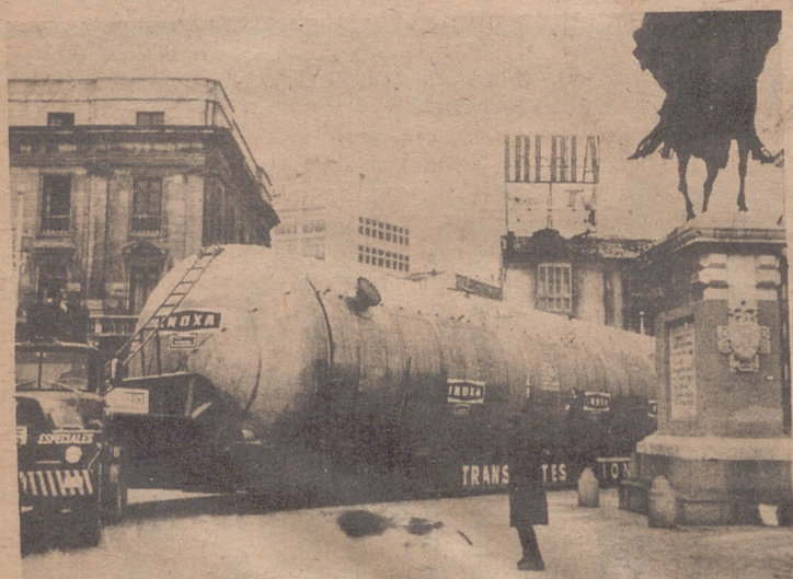
BURGOS.— Ante la estatua del Cid en la capital burgalesa circula el gigantesco transporte con un tanque de 5 metros de diámetro, 27 de longitud y un peso de sesenta y una toneladas, en acero inoxidable Aisi-316, y el espesor de la chapa en virolas de 10 mm. Ha sido construido en la factoría Inoxa del Polo Industrial de Burgos y va destinado a la planta de Tileno de Montoro en Puertollano. Se calcula que el transporte durará 25 días. (Foto Europa Press).
