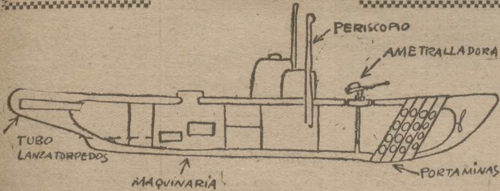
ESQUEMA Y CARACTERISTICAS DEL SUBMARINO ALEMÁN "U. C.-48".
