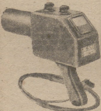
El detector nuclear de Geiger-Müller, cuya extraordinaria sensibilidad permite descubrir radiaciones atómicas por muy ocultas que se encuentren. El cañón de la pistola es una cámara de ionización sensible a los rayos X, gamma y beta, y la lectura de los mismos se hace fácilmente en miliamperios.
