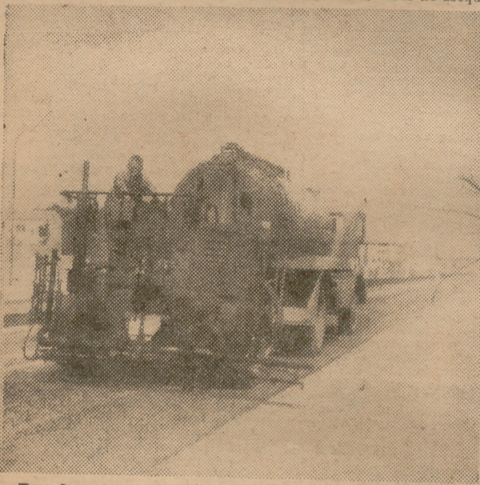
Tres fases de los trabajos de pavimentación de la nueva avenida de Albacete; en la primera, el betún asfáltico es pulverizado sobre la piedra tendida; en la segunda, los camiones de la empresa cargan automáticamente la gravilla mezclada con betún, y en la última, la máquina terminadora la distribuye sobre el suelo, creando una magnífica pista.
