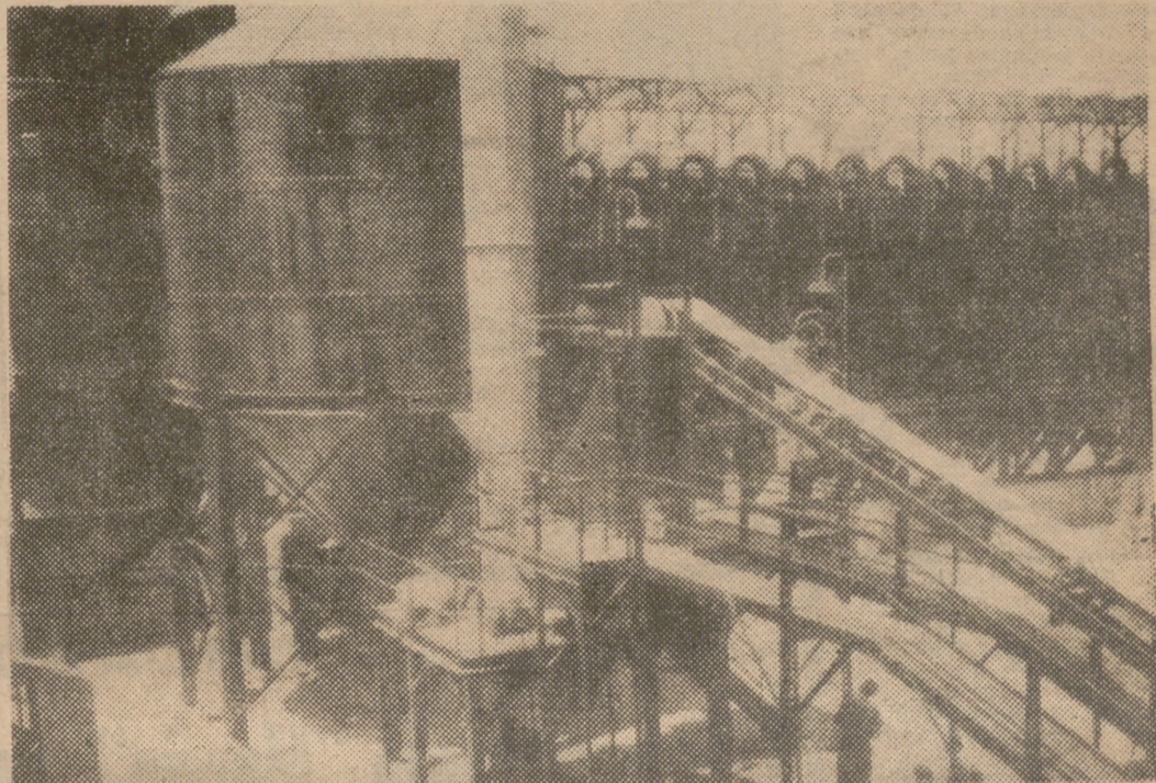
Hornos de destilación, recientemente instalados en las minas de azogue de Almadén y que han sido visitados hoy por Su Excelencia el Jefe del Estado. (Foto Gifra.)
