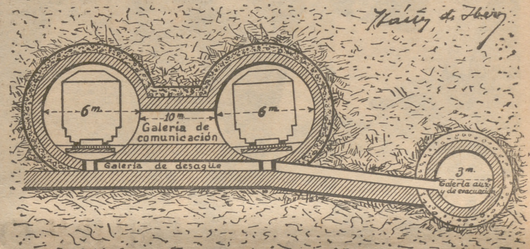
Sección transversal del proyectado túnel del Estrecho de Gibraltar, con sus galerías para ferrocarril en ambas direcciones y otra galería auxiliar y de evacuación
