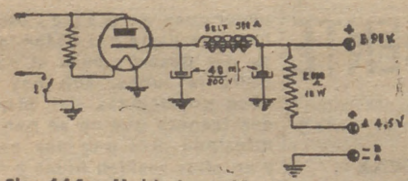
Fig. 114.—Unidad rectificadora mediante lámpara
