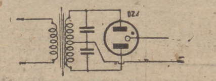
Fig. 105.—Célula de filtro
