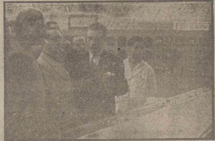
Sanz Orpio, acompañado del Consejo Económico Sindical, en su reciente visita a la central térmica de Compostilla. En la sala de mandos, el señor Grannell explica el funcionamiento de los pupitres de control y medida.
