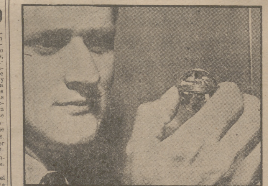
El doctor James M. Lafferty, de la General Electric, sostiene en la mano un pequeño receptor de radio, de su invención, y aplicable para inserción quirúrgica debajo de la piel de los perros en los experimentos de estimulación nerviosa sin dolor. El experimentador estimula el nervio mediante una señal radiada que el aparato recibe. El receptor tiene el tamaño de una pelota de ping-pong.
