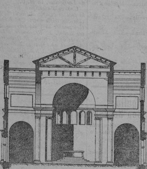
Sección transversal mirando al presbiterio
