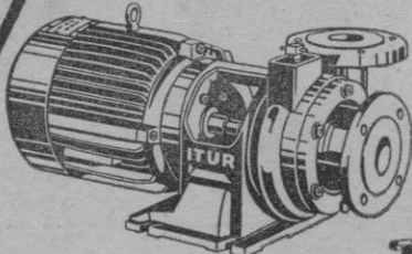
Electrobombas centrífugas monobloque y sobre bancada a base de motor y bomba independientes para caudales de hasta 3.600 m 3 /hora y alturas de 350 m. c. a.
