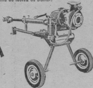
Bombas centrífugas eje libre y con multiplicador de velocidad para accionamiento por toma de fuerza de tractor.
