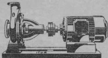
Electrobombas centrífugas monobloque y sobre bancada a base de motor y bomba independientes para caudales de hasta 3.600 m 3 /hora y alturas de 350 m. c. a.
