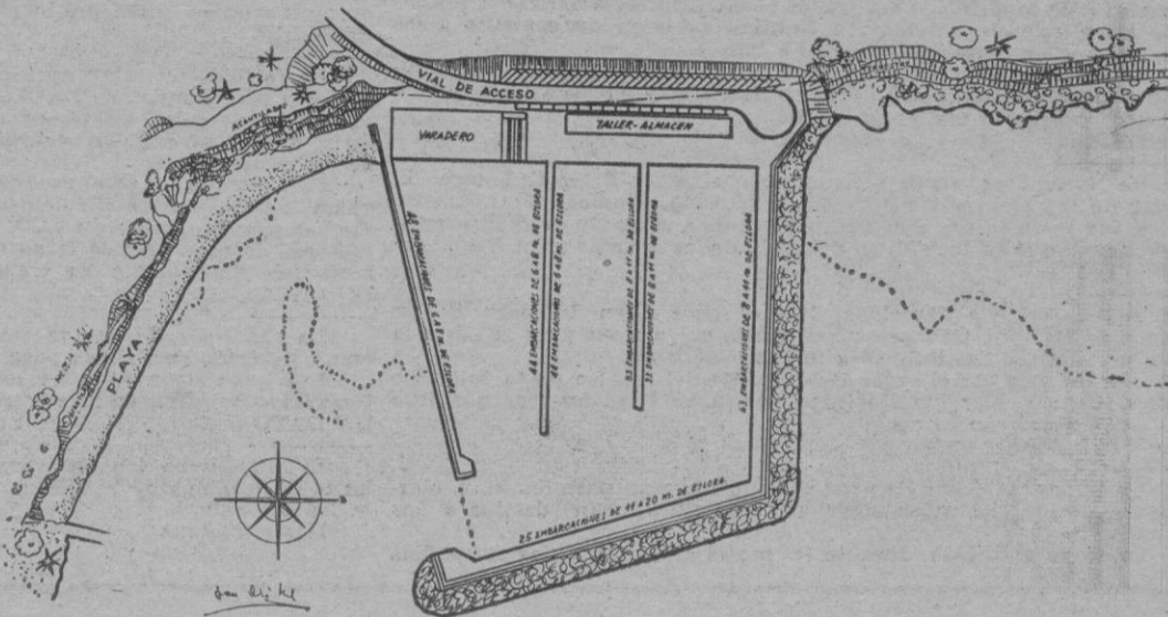
Este es el Puerto deportivo para 300 embarcaciones que se construirá en la Urbanización «El Toro» donde se edifica el chalet de la Cesta de Navidadde Baleares. El proyecto es del Ingeniero de Caminos, Canales y Puertos de nuestra ciudad, señor Cerdó.
