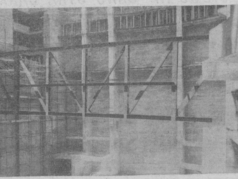
UN MOMENTO DEL IZAMIENTO DE LA VIGA DE CATORCE TONELADAS, YA A PUNTO DE SITUARSE EN SU LUGAR DEFINITIVO A CUARENTA METROS. ES UNA REALIZACION ARQUITECTONICA SIN PRECEDENTES EN NINGUNA EDIFICACION DE LAS EFECTUADAS EN LA ISLA. — (Foto Terrades.)
