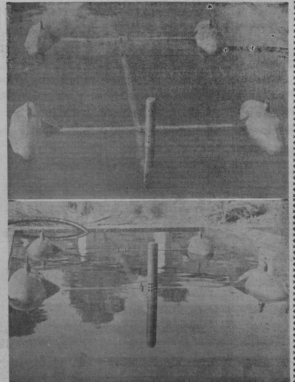
DOS ASPECTOS DEL APARATO INVENTADO POR EL SR. GIRONA, PARA VENCER LAS MANCHAS DE HIDROCARBUROS SOBRE EL MAR, TAN PELIGROSAS QUE PUEDEN LLEGAR A CONVERTIRSE EN TEMIBLES «MAREAS NEGRAS». LAS FOTOGRAFÍAS REVELAN PERFECTAMENTE LA EXPLICACION QUE NOS DA EL SR. GIRONA EN EL PRESENTE REPORTAJE. UN TUBO CONVENIENTEMENTE AGUIERADO Y QUE SE CONSIGUE MANTENER EN UNA POSICION SEMI-FLOTANTE, ASPIRA TODO LO QUE ESTE COLOCADO SOBRE LA SUPERFICIE DEL MAR.
