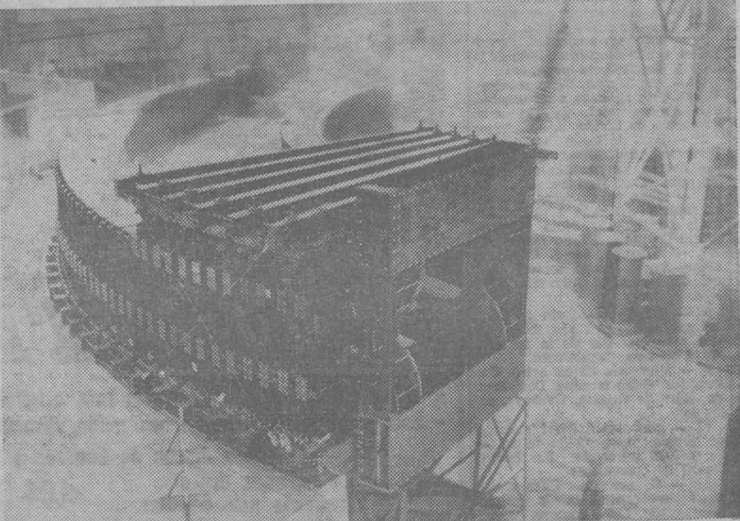
ESTE ES EL ACCELERADOR DE PARTICULAS DE BERKELEY (CALIFORNIA), QUE EN EL TIEMPO DE SU MONTAJE (1950) ERA EL MAS POTENTE DEL MUNDO CON SU CAPACIDAD DE ENERGIA DE 6 MILLONES DE ELECTRON-VOLTIOS. — (Foto Cifra)
