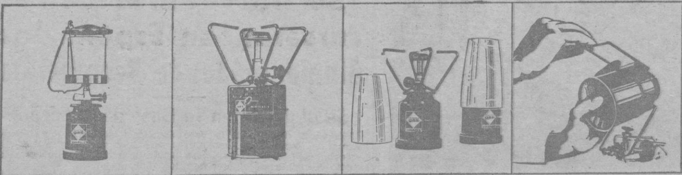
LUMOGAS "C" Altura: 30 cms. Diám.: 10 cms. MINIGAS "S" Altura: 20 cms. Diám.: 9 cms. MINIGAS "L" Altura: 24 cms. Diám.: 10 cms. Peso: 610 grs. Consumo: 20 a 30 grs. por h. Peso: 415 grs. Consumo: 50 grs. por hora. Peso: 580 grs. Consumo: 50 grs. por hora.
