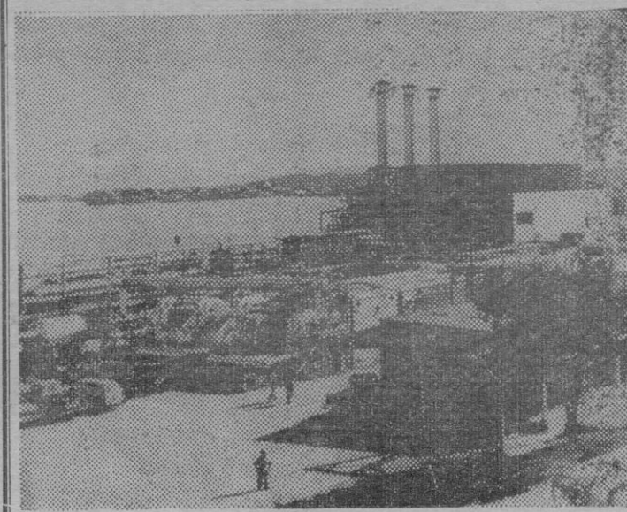
CASI DIEZ MILLONES DE LITROS DE AGUA DESTILADA «FABRICA» CADA DIA ESTA PLANTA INSTALADA EN GUANTANAMO. LA MATERIA PRIMA NO PUEDE AGOTARSE: ES EL ANCHO MAR. Y, DE PROPINA, PRODUCE 350.000 KILOWATIOS-HORA TAMBIEN POR DIA.
