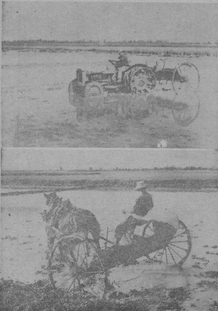
LA MAQUINA SEMBRADORA DE SEMILLAS DE ARROZ PUEDE MOVERSE POR TRACCION ANIMAL O MECANICA; COMO PUEDE OBSERVARSE EN LAS DOS FOTOGRAFIAS QUE ILUSTRAN EL TRABAJO. — (Foto Cifra)
