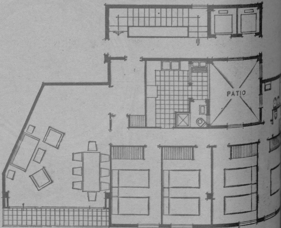
PLANTA PISO TIPO H
