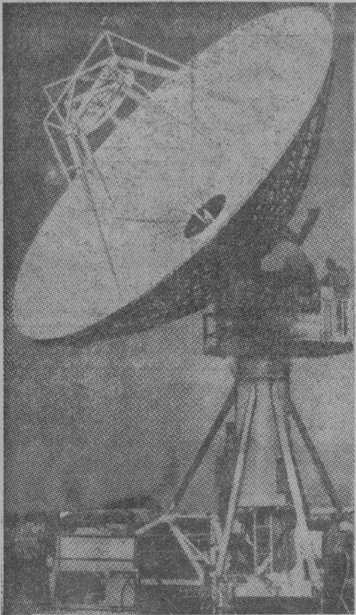
LA PRIMERA ESTACION TERRESTRE ALEMANA PARA LA TRANSMISION DE TELEFONEMAS, TELEESCRITO Y DATOS A TRAVES DE TODOS LOS SATELITES ARTIFICIALES DEL TIPO «TELSTAR» Y «RELAY» FUE INAUGURADA RECIENTEMENTE LA INSTALACION CONSISTE EN UNA ANTENA DE ESPEJOS PARABOLICOS DE UN DIAMETRO DE NUEVE METROS Y EN UN REMOLQUE PARA TRACTORES-ALBARDA, EN QUE ESTA INSTALADO EL SISTEMA DE CONTROL Y DE GOBIERNO.
