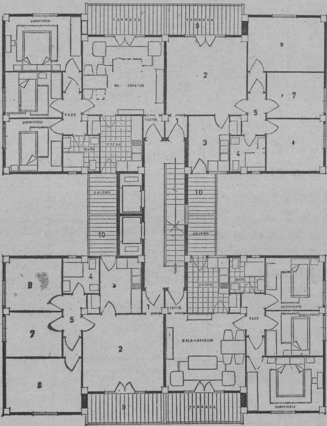
PLANTA "BLOQUE C"
