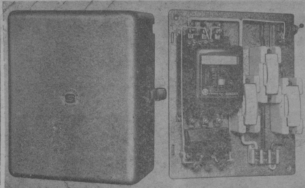
Maniobra EPM, para la puesta en marcha y protección de motores eléctricos.
