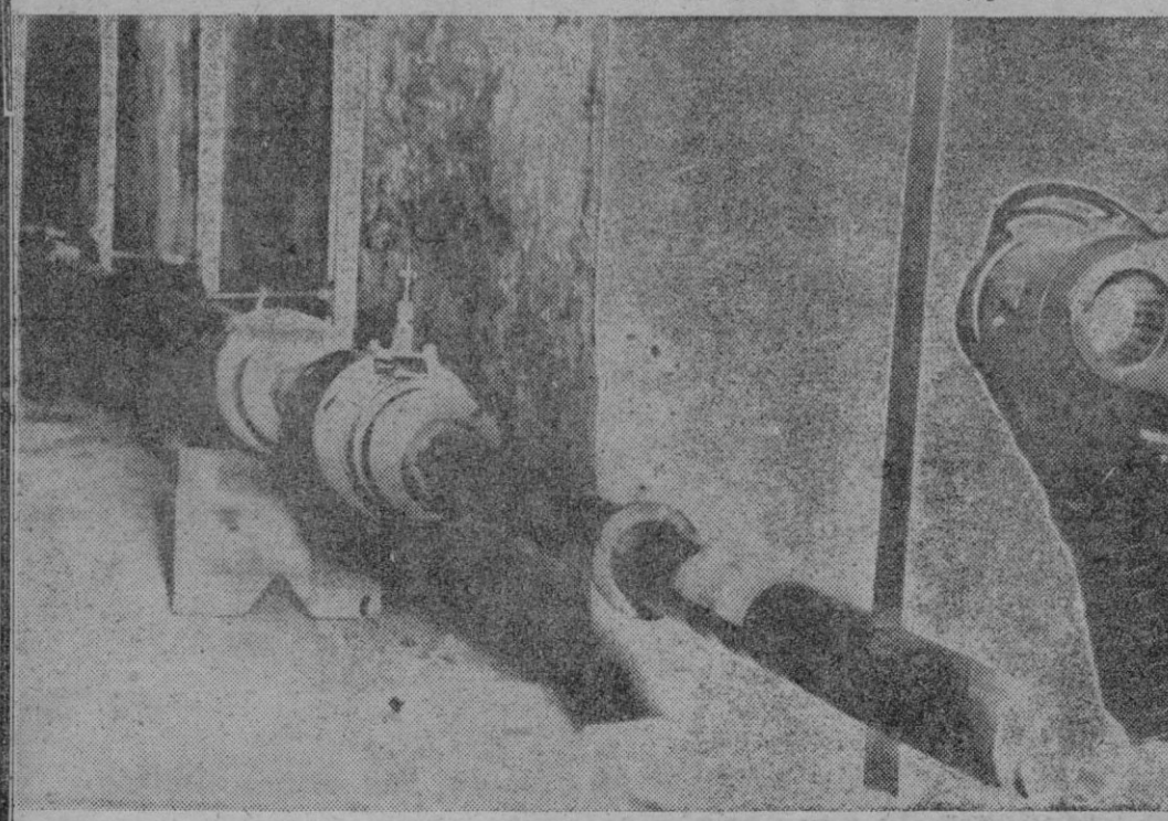
PARIS. — ESTE SUPERCABLE TELEFONICO DE 9 CM. DE DIAMETRO, PUEDE TRANSMITIR PERFECTAMENTE ALREDEDOR DE 200.000 COMUNICACIONES SIMULTANEAS.—(Foto CIFRA)
