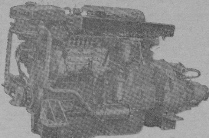
MD 47 B - DIESEL, DESDE 83 A 200 H.P. CON CAMBIO DE MARCHAS Y REDUCTORA.
