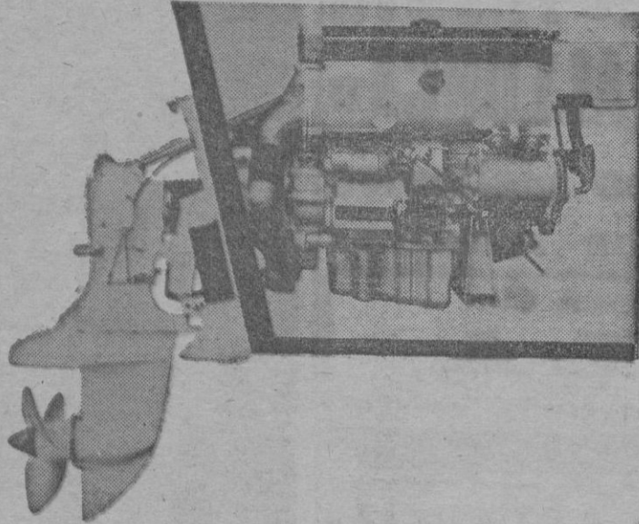
EL NUEVO «AQUAMATIC» DIESEL EN CUATRO Y SEIS CILINDROS DE 60 y 85 H.P.
