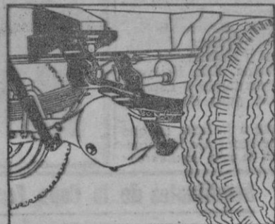
PUENTE TRASERO DE COJINETES CONICOS Y PALIERES FLOTANTES.
