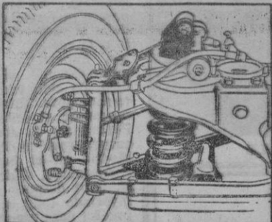
SUSPENSION DELANTERA A DOBLE EFECTO
