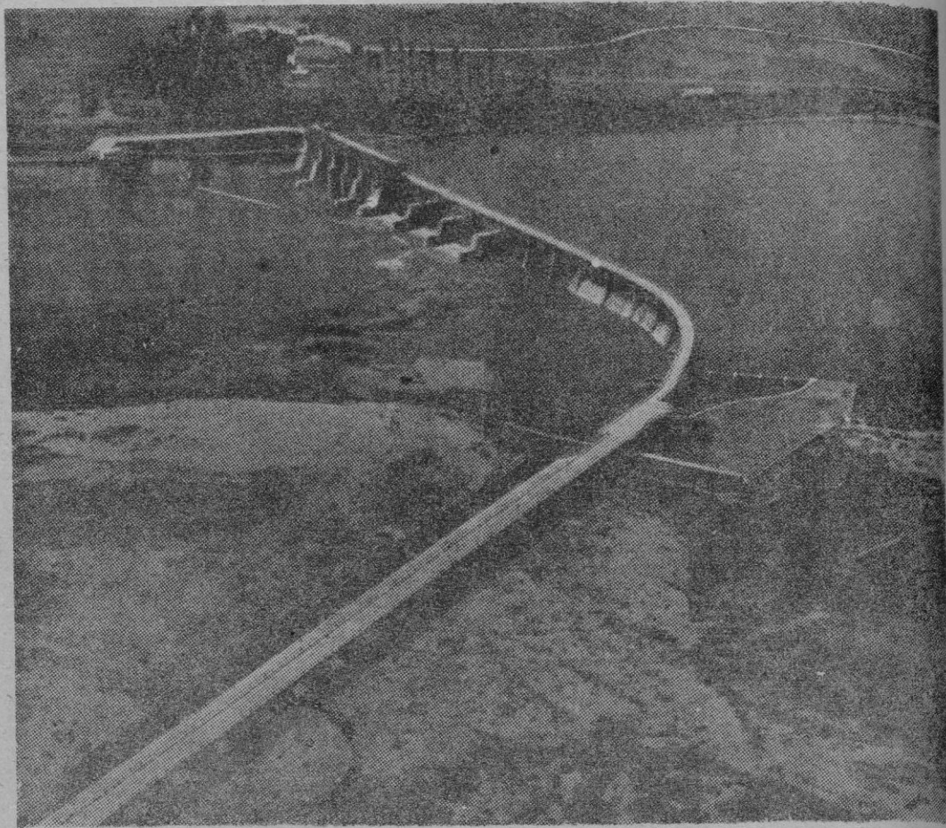
Fotografía aérea del conjunto de la presa de Montijo, apreciándose los distintos tipos de compuertas y las tomas de los canales de Montijo y Lobón. Esta es una más de las realizaciones del Plan Badajoz.
