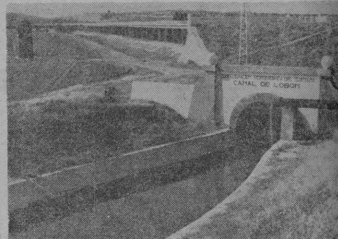
Kilómetros y más kilómetros de acequias se construyeron para el regadío. El canal de Lobón alimenta a muchas de ellas.
