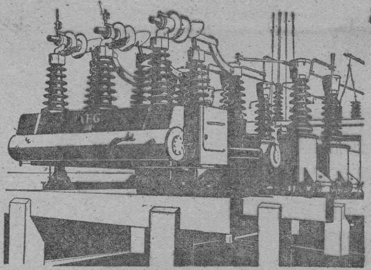
Interrupor de aire comprimido para 65.000 Voltios - 1.000 Amperios, capacidad disruptiva: 1.500.000 KVA
