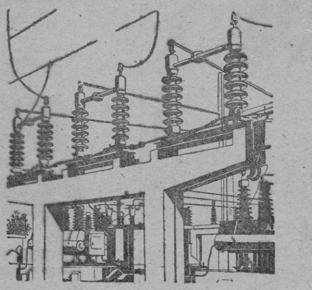
Seccionador tripolar para 66.000 Voltios, 600 Amperios
