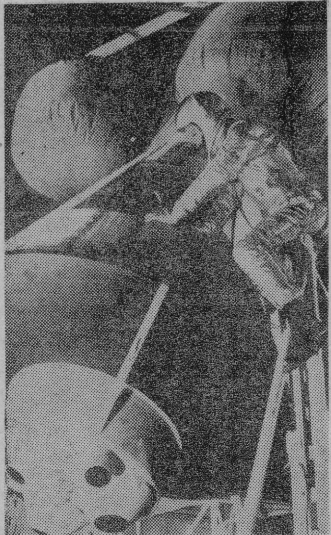
Esta es la última versión de un vehículo para mandar a un hombre al espacio. En la foto se ve al piloto en el momento de entrar en el vehículo y, en la parte superior de la misma, dos depósitos de aire que permitirán que el vehículo flote cuando llegue al agua.
