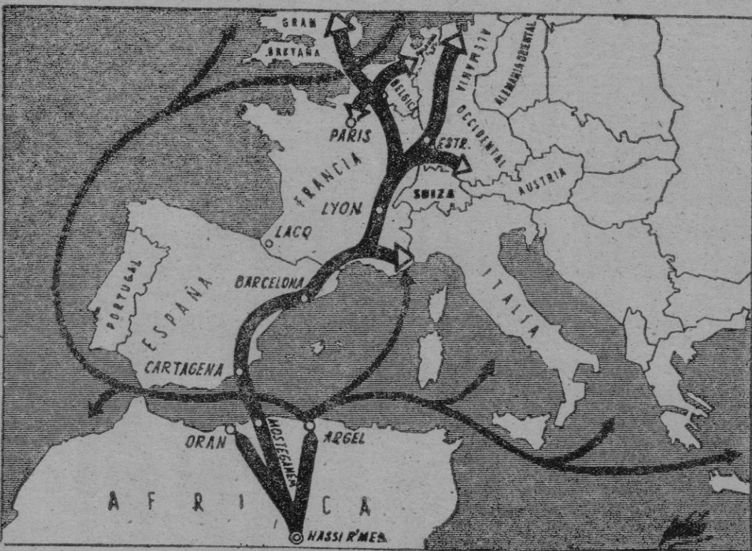
El gráfico indica en trazo ancho el camino que seguirá el gaseoducto entre los campos petrolíferos y de gas del Sahara francés hasta el cabo de Palos, cruza el Mediterráneo por conducción submarina. Después continúa por la costa levantina española, atraviesa Barcelona y penetra en Francia. Desde este país podrán construirse otras líneas en dirección a Italia y al centro europeo. El gas será almacenado a su llegada a Francia en depósitos naturales o artificiales. La línea delgada indica las posibles rutas marítimas, partiendo de Argel, para el transporte a Europa del gas natural del desierto. Ello obligaría a una licuación del metano, principal elemento del gas. Esta operación es muy costosa y por ello se ha decidido la construcción del gaseoducto que atravesará España.
