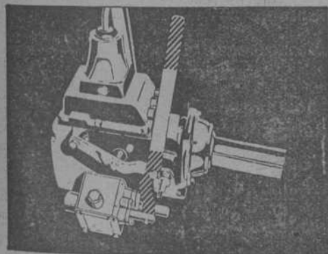
Caja de cambios de cuatro velocidades, que aumenta el rendimiento del camión. A la caja de cambios se puede acoplar una toma de fuerza para aplicarla a cualquier uso industrial.
