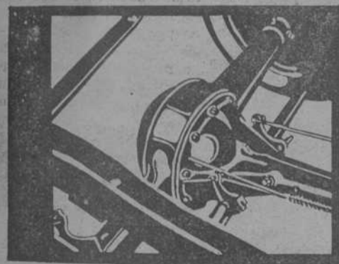
El nuevo eje trasero está encerrado en una sólida cubierta, provista de una tapa, que permite inspeccionar y ajustar el eje sin desmontarlo.
