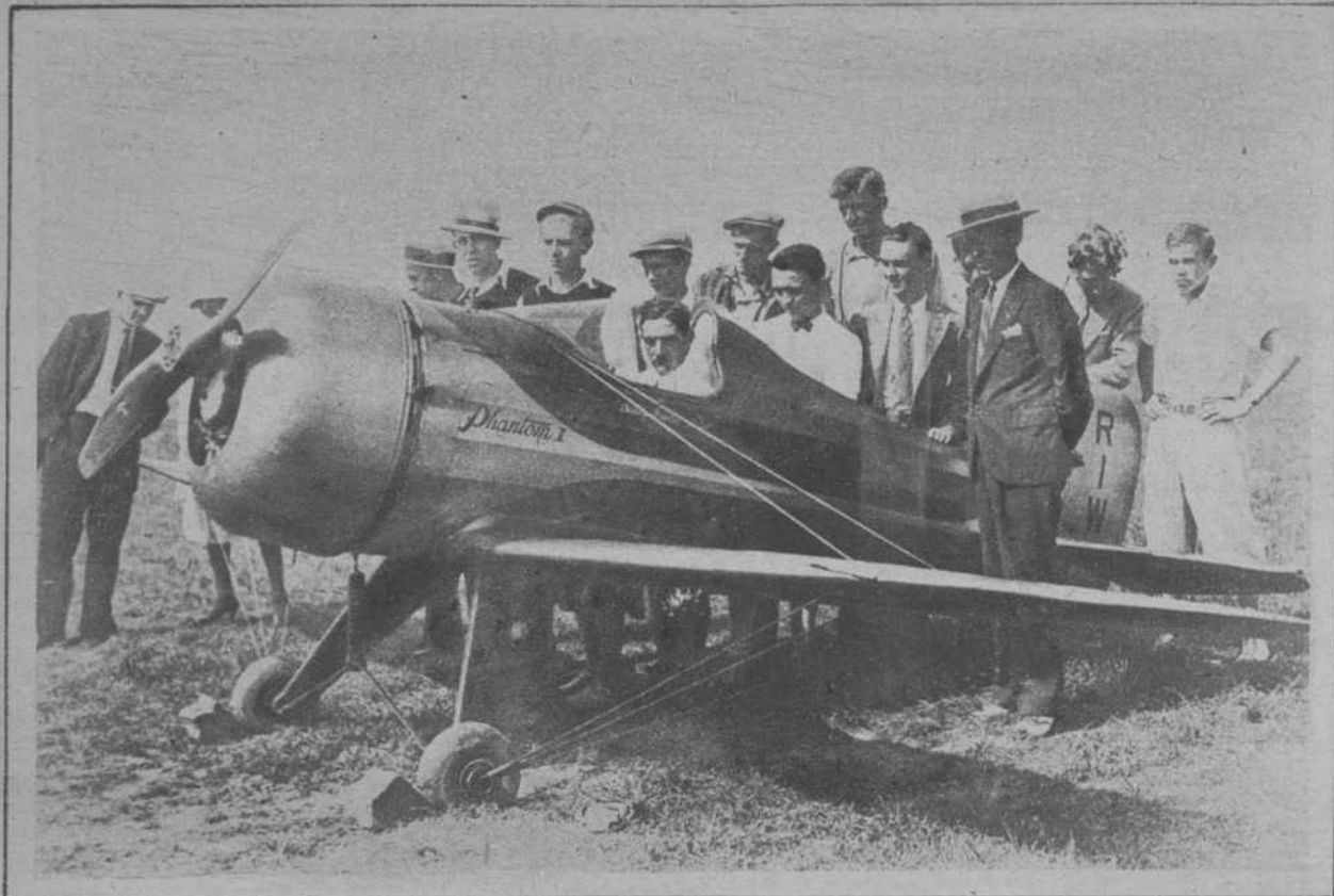
El aviador Danny Fowle, con su misterioso aeroplano «Phantom I», que por sus dimensiones y detalles técnicos, ha llamado la atención en el concurso celebrado estos días en Chicago. Pesa el aparato 335 libras, tiene una altura de 12 pies y sus motores desarrollan una fuerza de 72 HP. — (Fot. Keystone)
