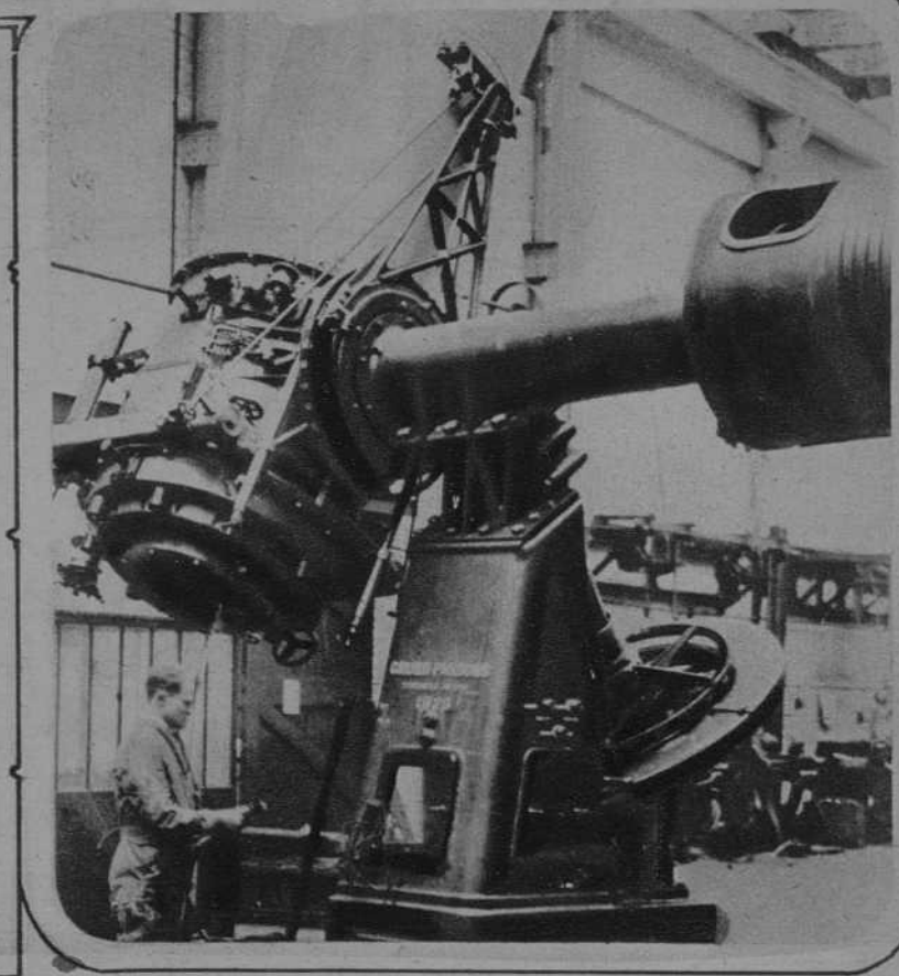
El mayor telescopio de Inglaterra, construido para el Observatorio de Hedimburgo
