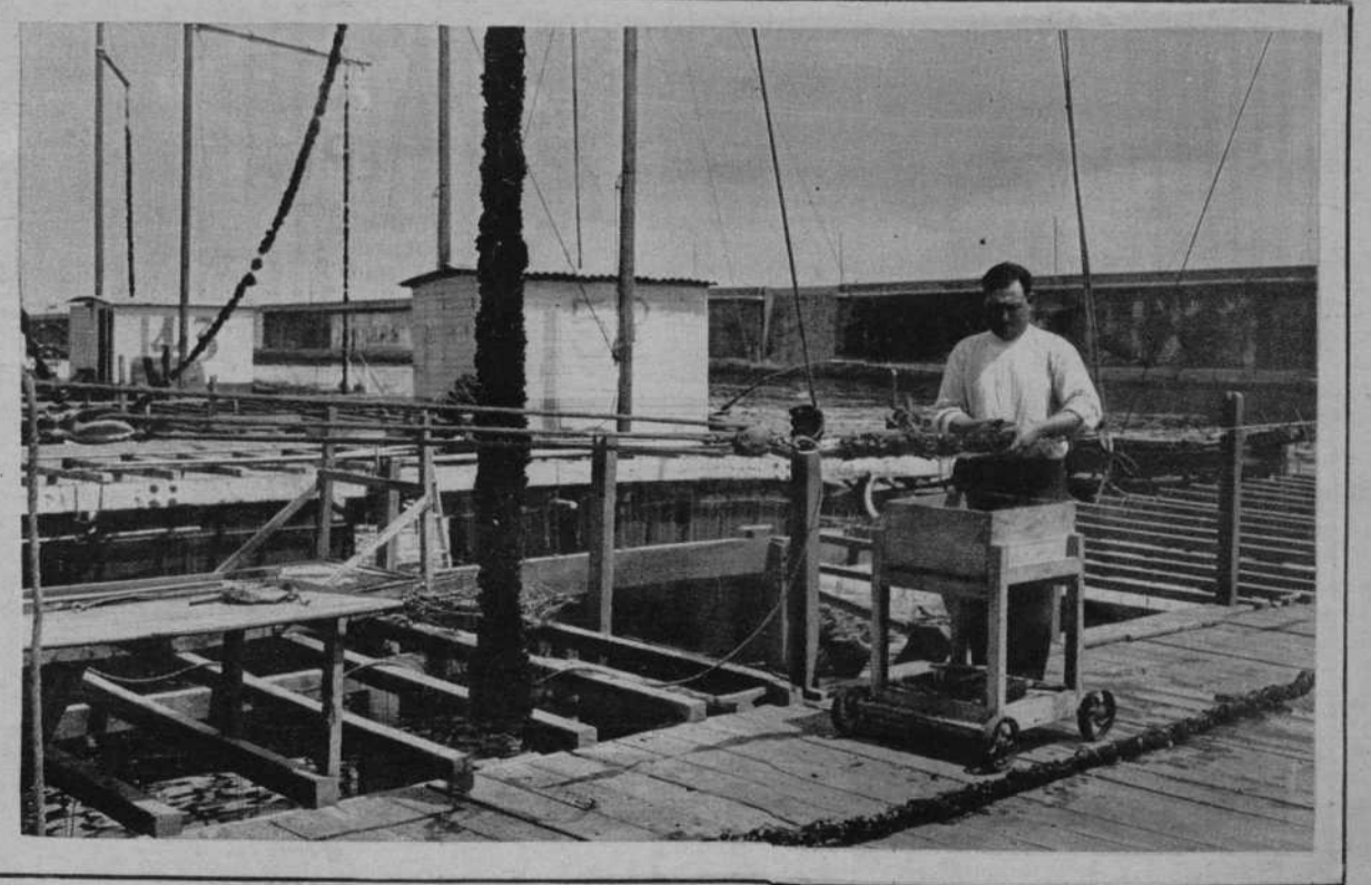
...Un alambre con puntas como de espino, de trecho en trecho; alrededor de él se van colocando los mejillones de cría, envolviéndolos a modo de bolsa con una red que a medida que se enrolla se clava en los puntos salientes del alambre quedando sujeta...
