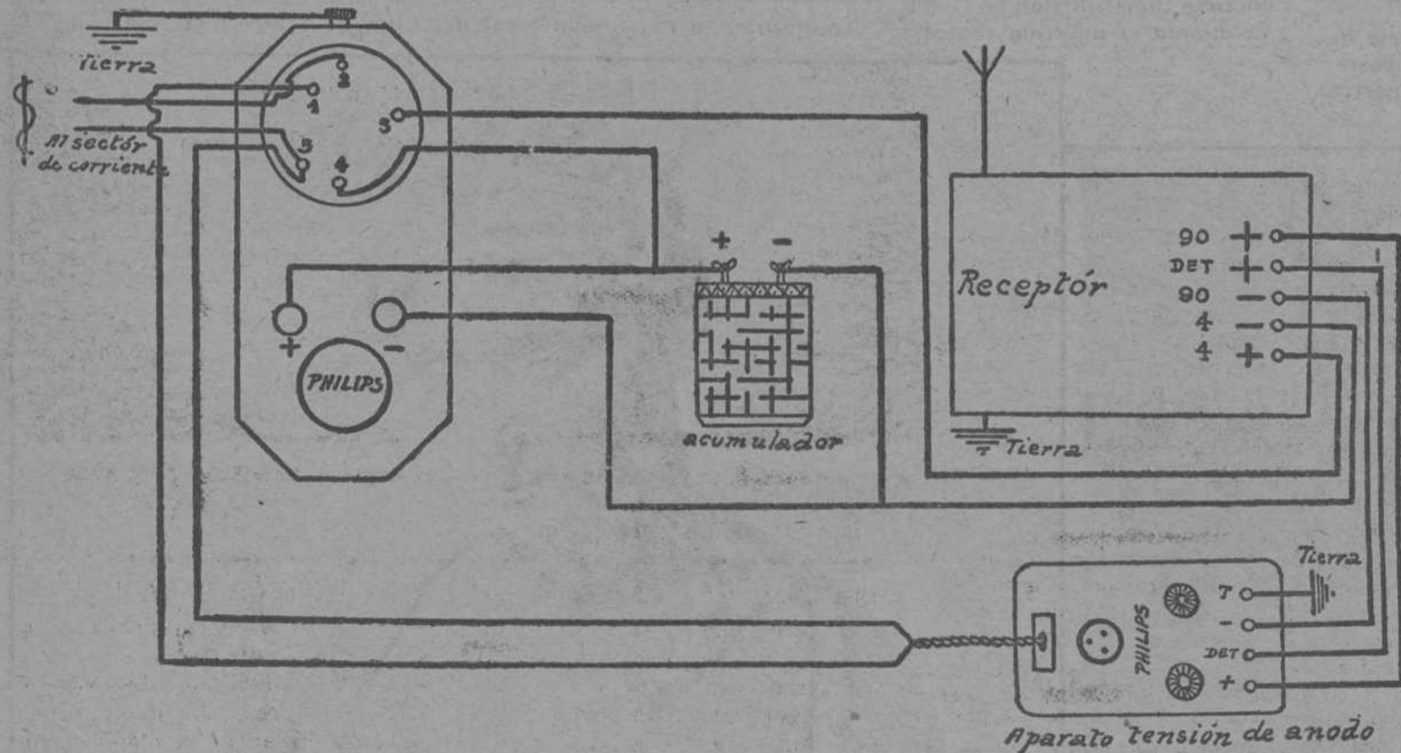
Esquema de conexión del rectificador «Miniatura», tipo 1017 con aparato receptor, acumulador y aparato de tensión de ánodo
