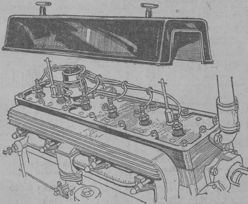
El cárter protector de las bujías y de la distribución que le da al motor «Citroën Six» el aspecto de una «válvula a la culata»
