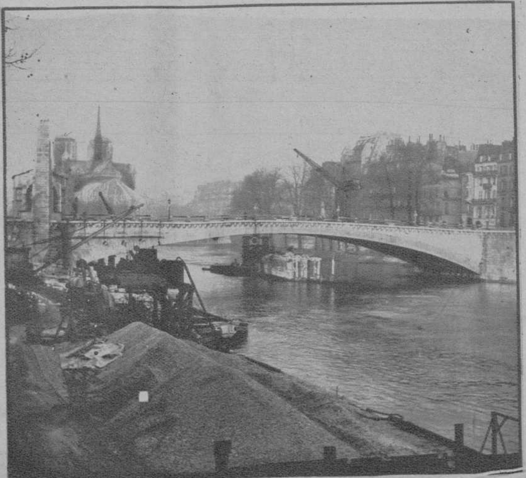
PARIS.—Nuevo puente sobre el Sena, construido en cemento armado. A la izquierda se colocará la estatua de Santa Geneveva, patrona de Paris. (Fot. Consorcio).
