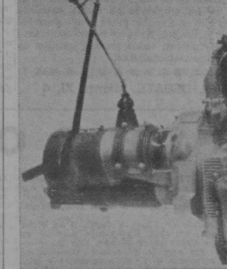
Un motor Diessel-Krupp de 60 HP., refrigerado por aire
