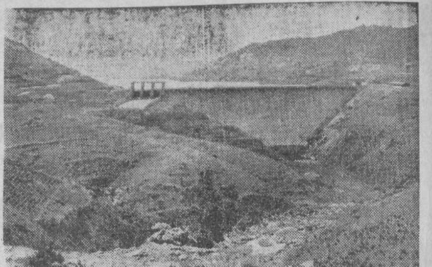
SALTOS DEL ALBERCHE.—La magnífica Presa de Burguillo, de 90 metros de altura y 300.000 m 3 de hormigón, que será visitada el próximo domingo por nuestros excursionistas.
