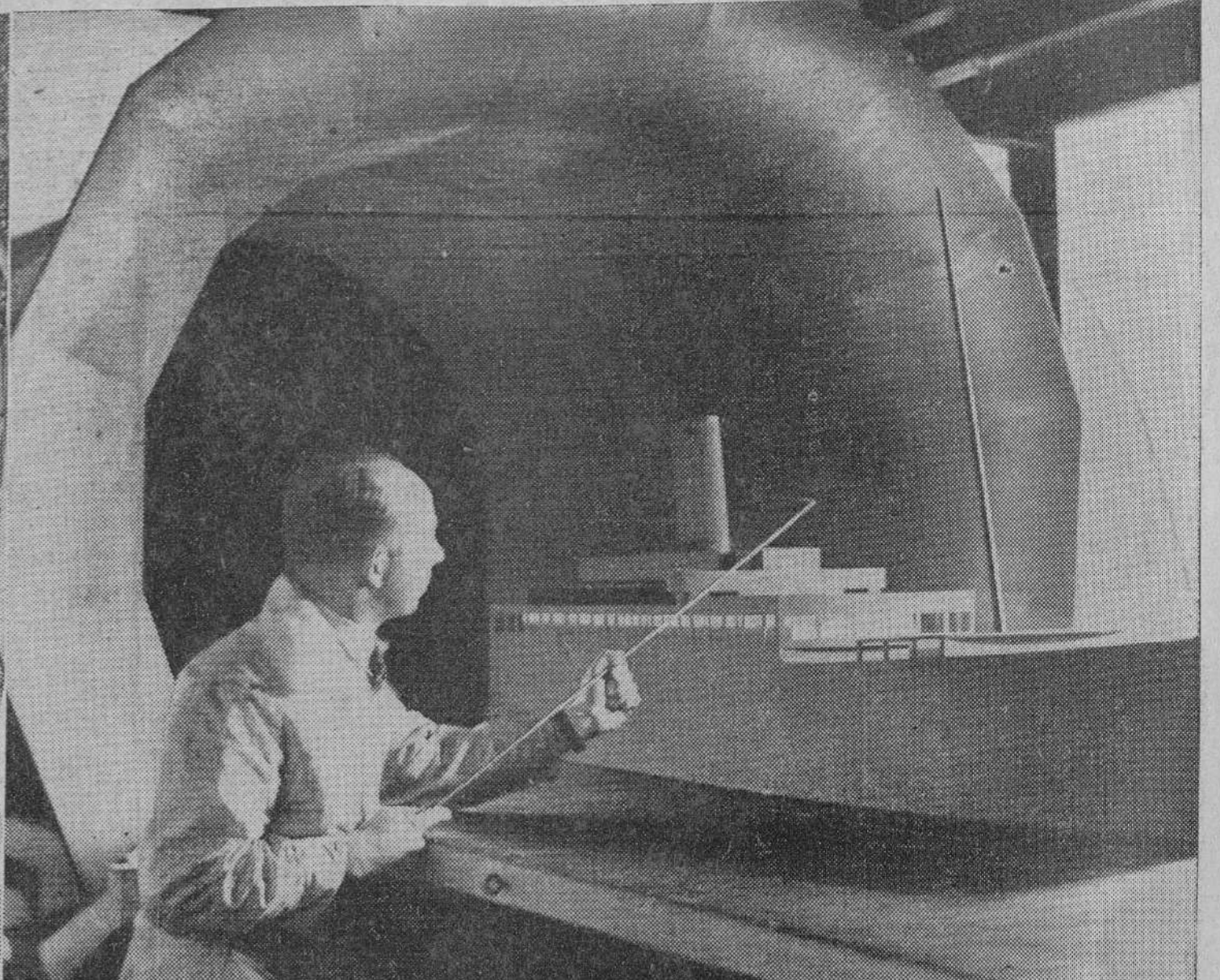
Modernamente se piensa que la forma de la parte del casco que sobresale de la línea de flotación, influye en la velocidad del navío. Los alemanes han montado en Hannover este túnel aerotécnico para hacer pruebas con maquetas de buques
