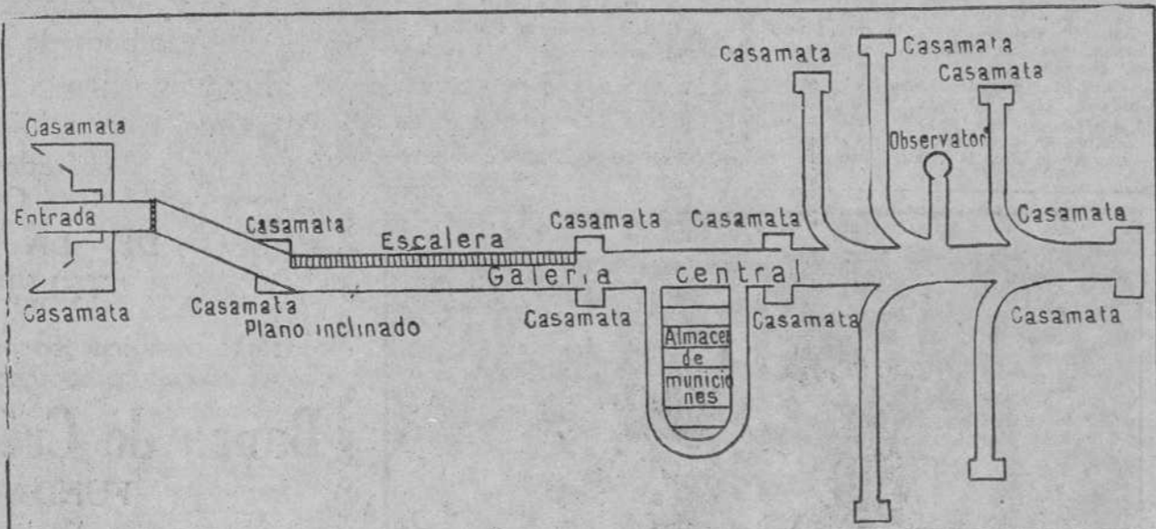
Esquema aproximado de una obra subterránea
