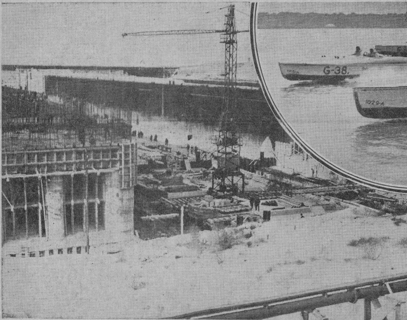
Una vista de la esclusa de nueva construcción del puerto de Dunkerque. Tiene una longitud de 280 metros por 40 de ancho
