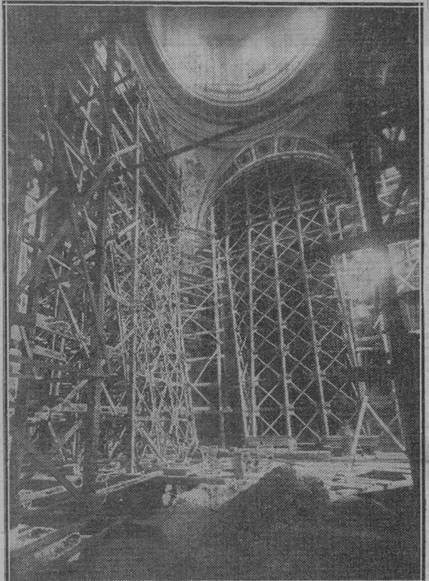
Armadura de hierro que en las obras de consolidación del Pilar ejecuta Zaragoza Industrial, S. A.
