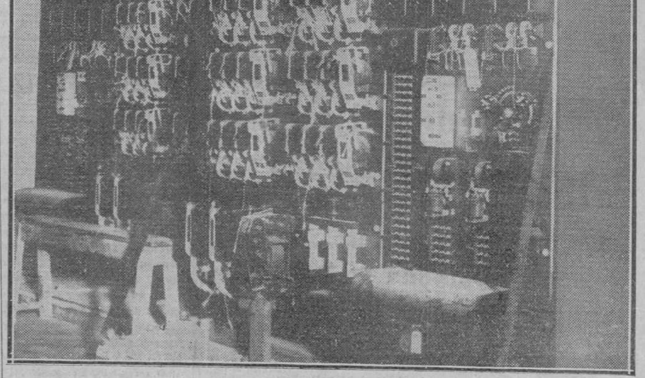
Cuadros eléctricos de mando desde los cuales se acciona todo el movimiento de la rotativa y que van encerrados en una cabina especial
