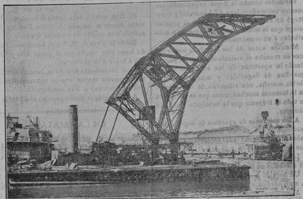
Ferrol: Grúa flotante elevando desde tierra una turbina de 62 toneladas para el «España».
