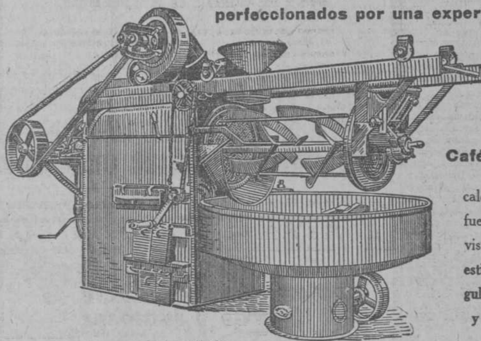
"METEOR" con mezclador estirado
