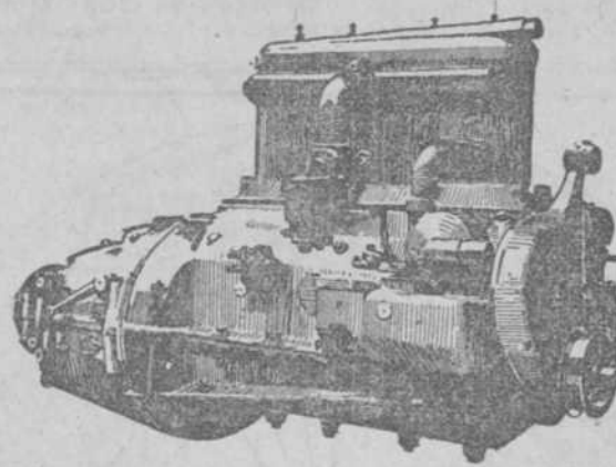
El bloque motor Panhard, sin válvulas, 16 H. P.
