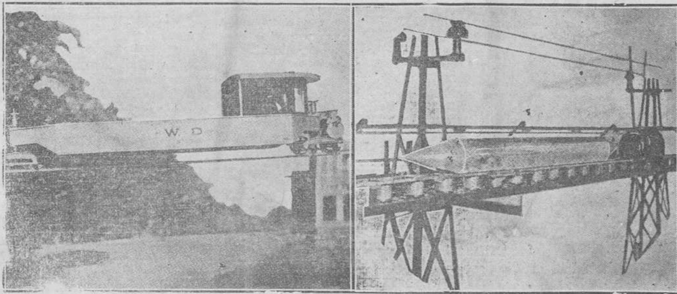
(6) El monoriel, con coches "Breman" equilibrados, en otro paso más hacia velocidades extraordinarias. Aquí se ve corriendo sobre un cable de alambre, única "vía" que necesita. (8) Vagón-torpedo para correspondencias tal como funciona en el modelo de línea experimental construido por Mr. Bachelet. Debido a que su sistema elimina toda la fricción se obtienen velocidades asombrosas.
