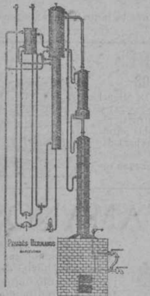
Aparato destilación continua á fuego directo. Producción del alcohol de 95 á 96°, ó sean 40° Cartier.
